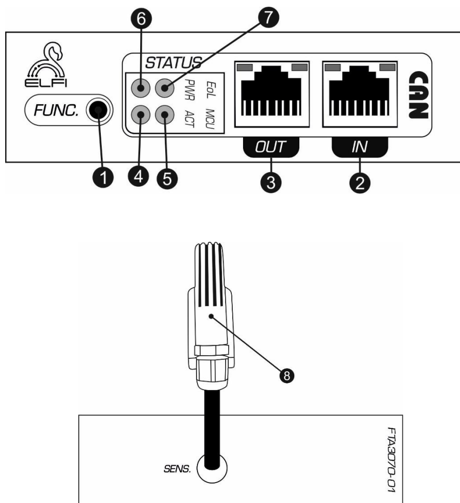
شکل ۲: نمای جانبی Node دما و رطوبت
