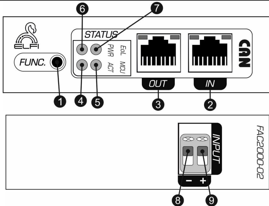
شکل ۲: نمای جانبی Node جریان DC
