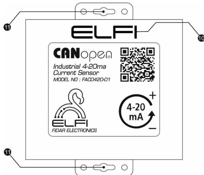
شکل ۳: نمای روبه روی Node ۲۰-۴ میلی آمپر تک کانال
