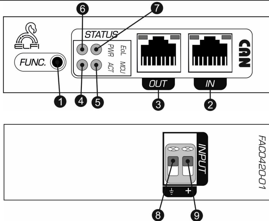
شکل ۲: نمای جانبی Node ۲۰-۴ میلی آمپر تک کانال
