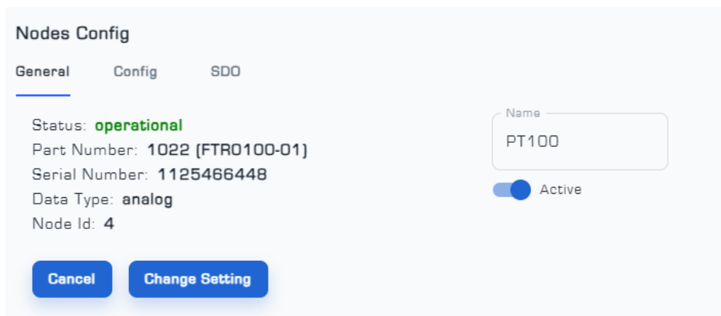
شکل ۵: منوی General از صفحه ی تنظیمات Node
