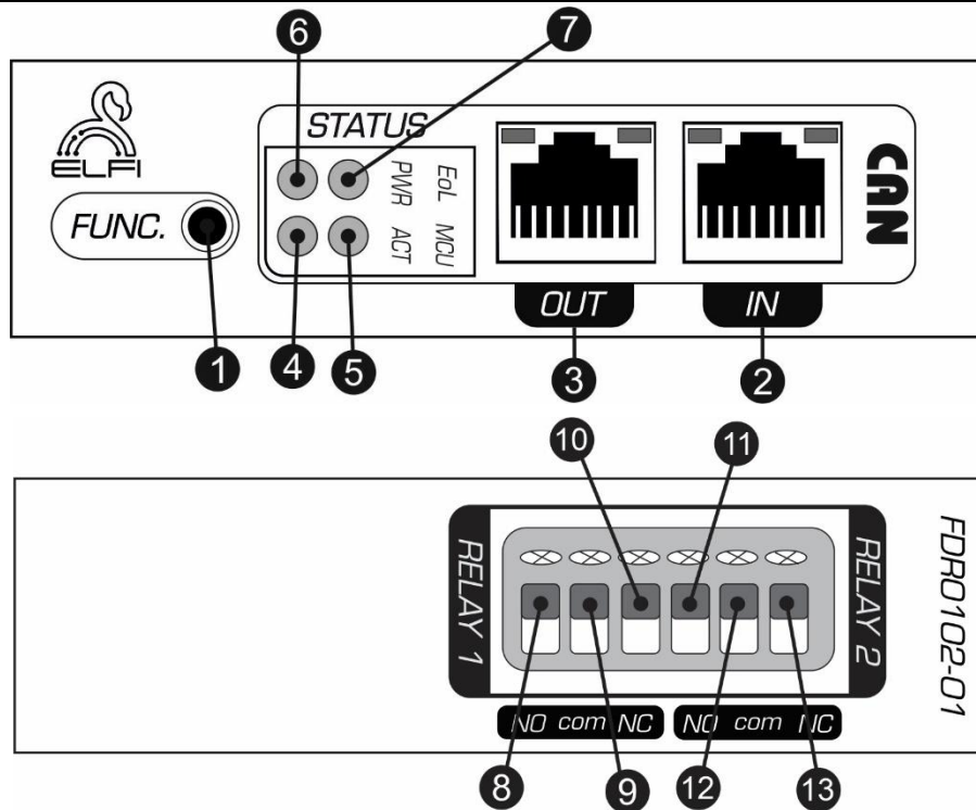
شکل ۲: نمای جانبی Node رله‌ی دوکانال
