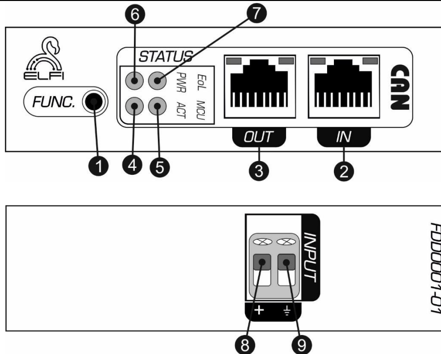
شکل ۲: نمای جانبی Node کنتاكت خشک تک کانال
