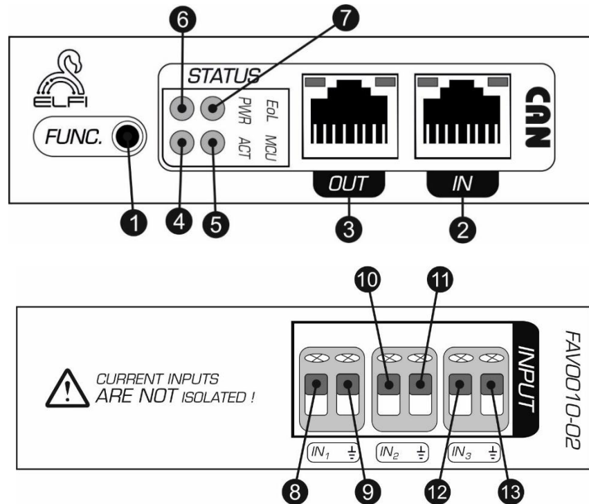
شکل ۲: نمای جانبی Node سطح ولتاژ مستقیم سه کانال
