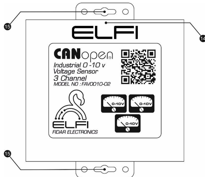
شکل ۳: نمای روبه روی Node سطح ولتاژ سه کانال
